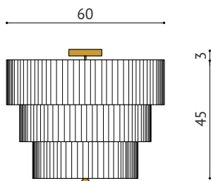
MODEL II WIDOK Z PRZODU
