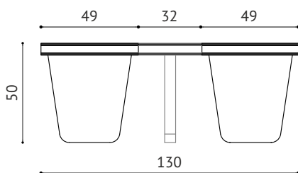
WIDOK Z BOKU (jednego modułu)
